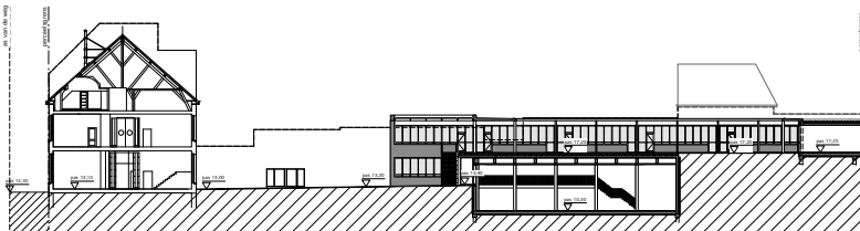
NIEUWE INPLANTING
