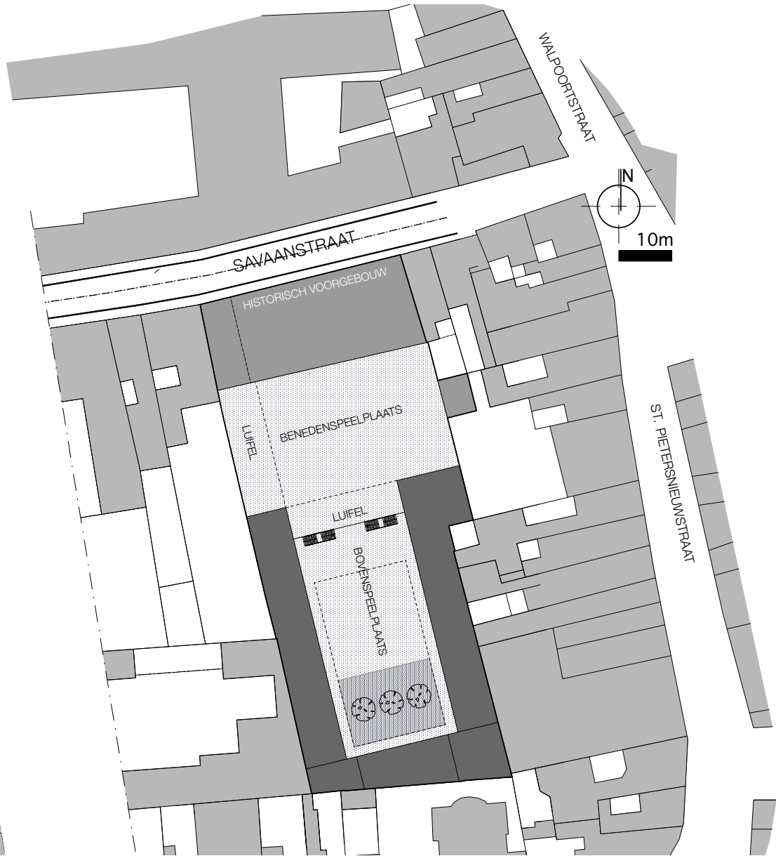
NIEUWE INPLANTING
